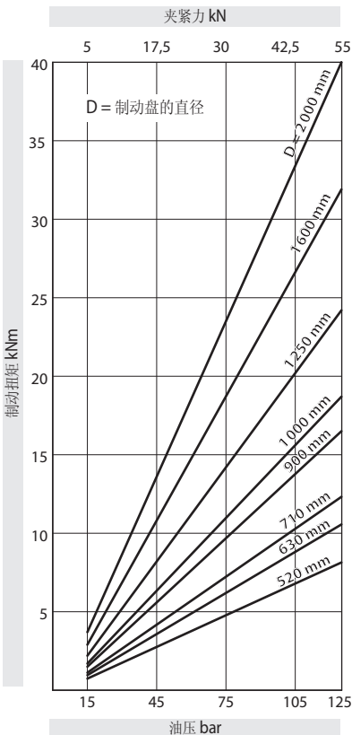
图表所示制动扭矩基于理论摩擦系数0,4。
